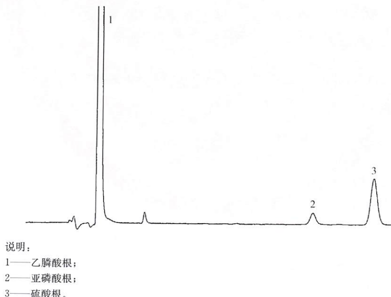
图 2 测定亚磷酸盐的三乙磷酸铝可湿性粉剂离子色谱图
